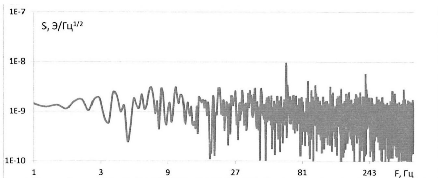
Рис. 8. Спектральная плотность магнитных шумов сенсора в диапазоне частот 1 – 500 Гц.
