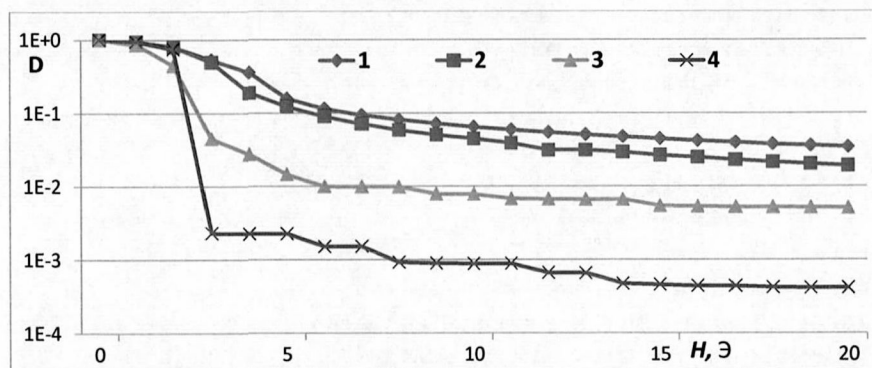
Рис. 7. Зависимость фактора деполаризации от величины насыщающего поля в плоскости для дисков: 1-одноступенчатый с вертикальным краем, 2-одноступенчатый с наклоном 45 градусов, 3-пятиступенчатый с наклоном 45 градусов, 4-непрерывный эллиптический профиль.
