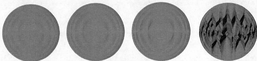
Рис. 6. Распределение намагниченности для пятиступенчатого диска при последовательном уменьшении внешнего магнитного поля, слева направо – 20 Э, 10 Э, 5 Э, 2,5 Э.
