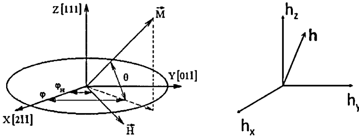
Рис. 1. Пленка феррит-граната во вращающемся в плоскости (111) магнитном поле H
