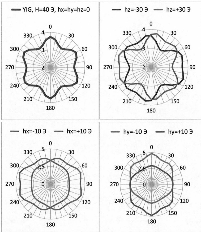
Рис. 2. Измеренные угловые зависимости магнитной восприимчивости в плоскости пленки \chi'(\varphi) в насыщающем поле H=40 Э и различных постоянных полях h_x , h_y и h_z , для феррит-граната Y_3Fe_5O_{12} .
