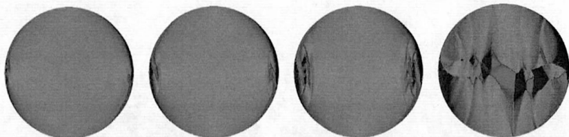
Рис. 5. Распределение намагниченности для одноступенчатого диска при последовательном уменьшении внешнего магнитного поля, слева направо – 20 Э, 10 Э, 5 Э, 2,5 Э.
