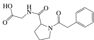
N-фенилацетил-L-пролилглицин
