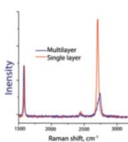
Рамановский спектр
