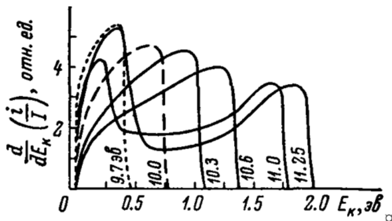
Рис. 1. Распределение электронов по кинетическим энергиям при фотоионизации бензола. Кривые приведены к одной интенсивности света.
