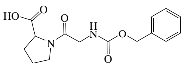
N-бензилоксикарбонил-глицил-L-пролин
