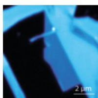
Интенсивность G-диапазона
