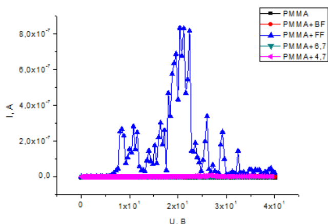
Рис. 1. Вольт-амперная характеристика структуры Al/ПММА+Доп/Al: 1–ПММА; 2–ПММА+БФ; 3– ПММА+ФФ; 4– ПММА+6,7; 5– ПММА+4,7.
