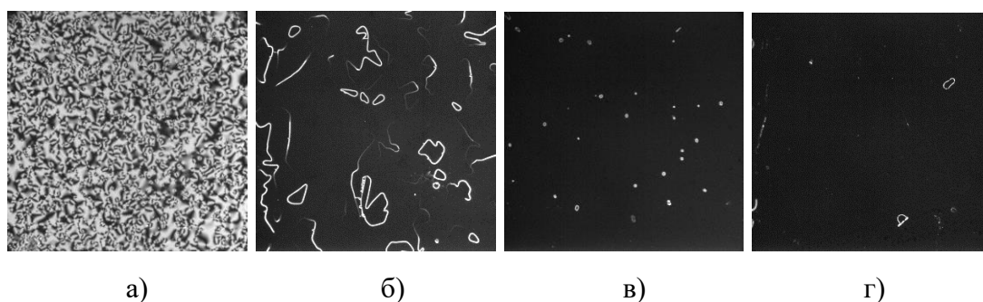
Рис. 1. Микроскопические изображения слоев МББА в геометрии скрещенных поляризаторов: а) 1 мин засветки ПВЦ, б) 7 мин, в) 15 мин, г) 30 мин.
