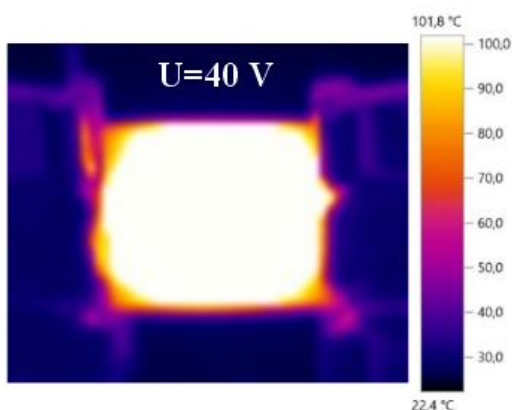
Рис.1. Термограмма полимерного композита на основе RG-P1.
